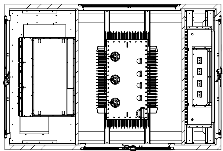
SECTION J-J SCALE 1 : 40
