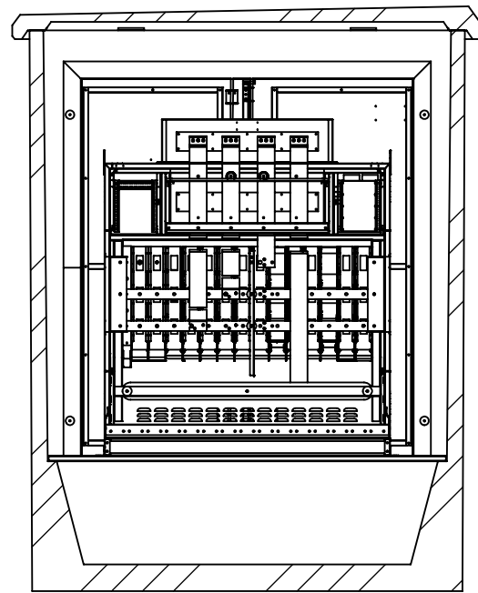
SECTION I-I SCALE 1 : 40
